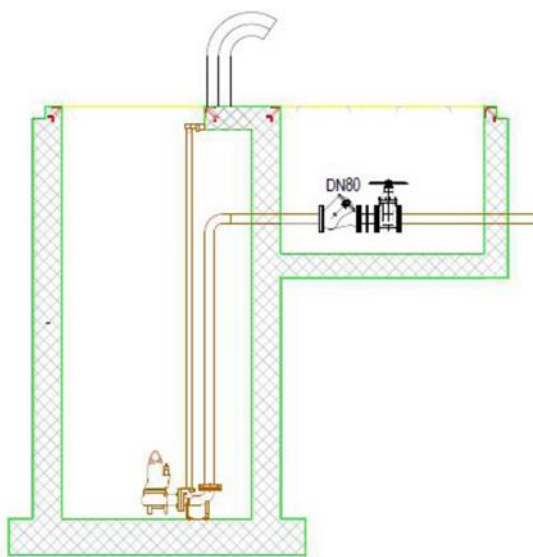
Slika 3.4. Presjek kroz objekat komore
