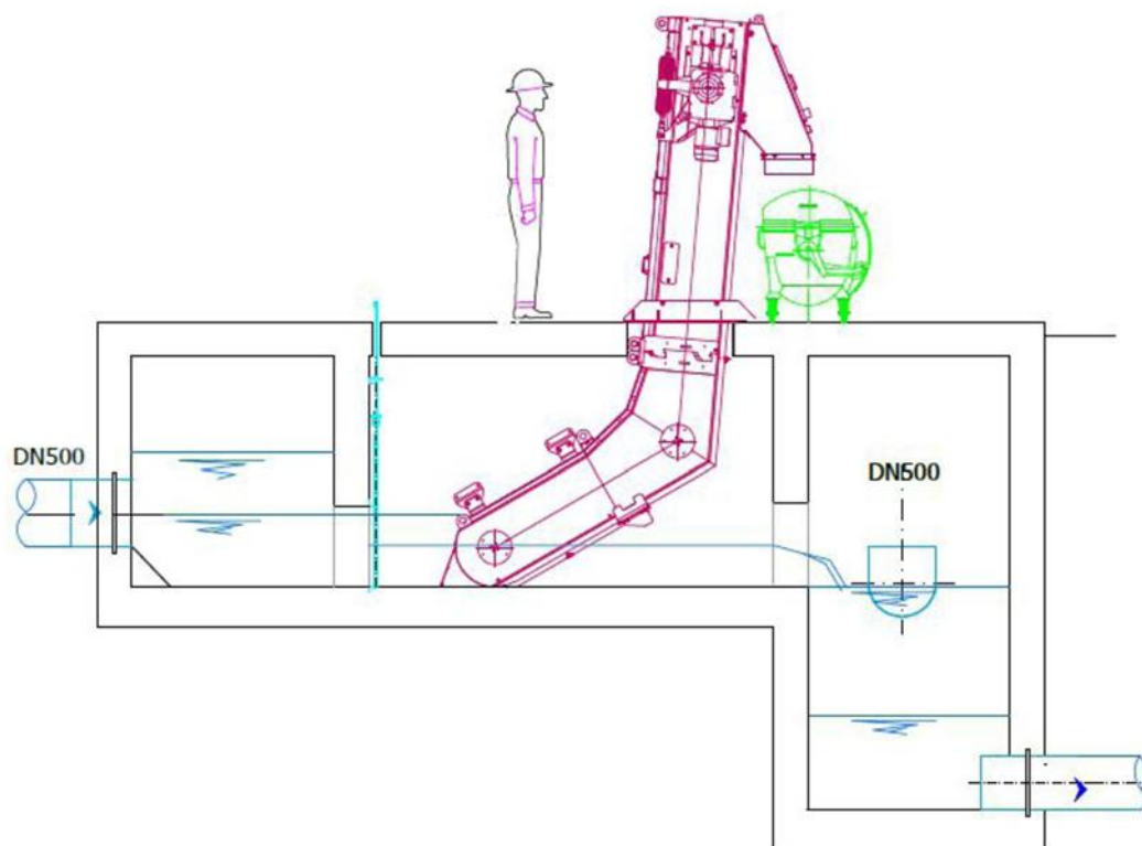
Slika 3.6. Presjek kroz prijemni šaht
